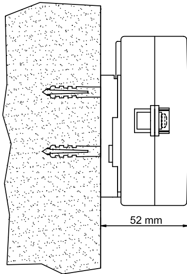
Boční pohled MULTICAL® 601 umístěný na zdi
