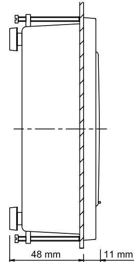
Boční pohled na MULTICAL® 601 namontovaný do panelu
